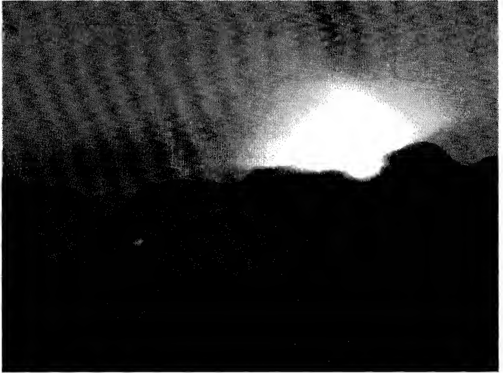
«فالق الإصباح» الشمس في حالة الشروق
